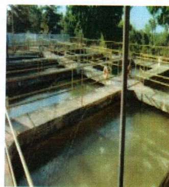
Decantação
