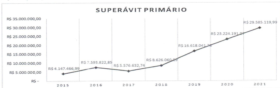
Gráfico 3: Superávit primário
